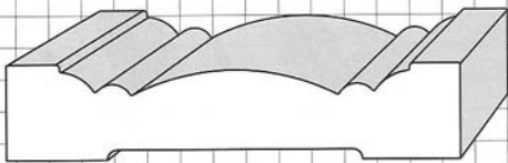
WM2013 3/4" x 3-9/16"
